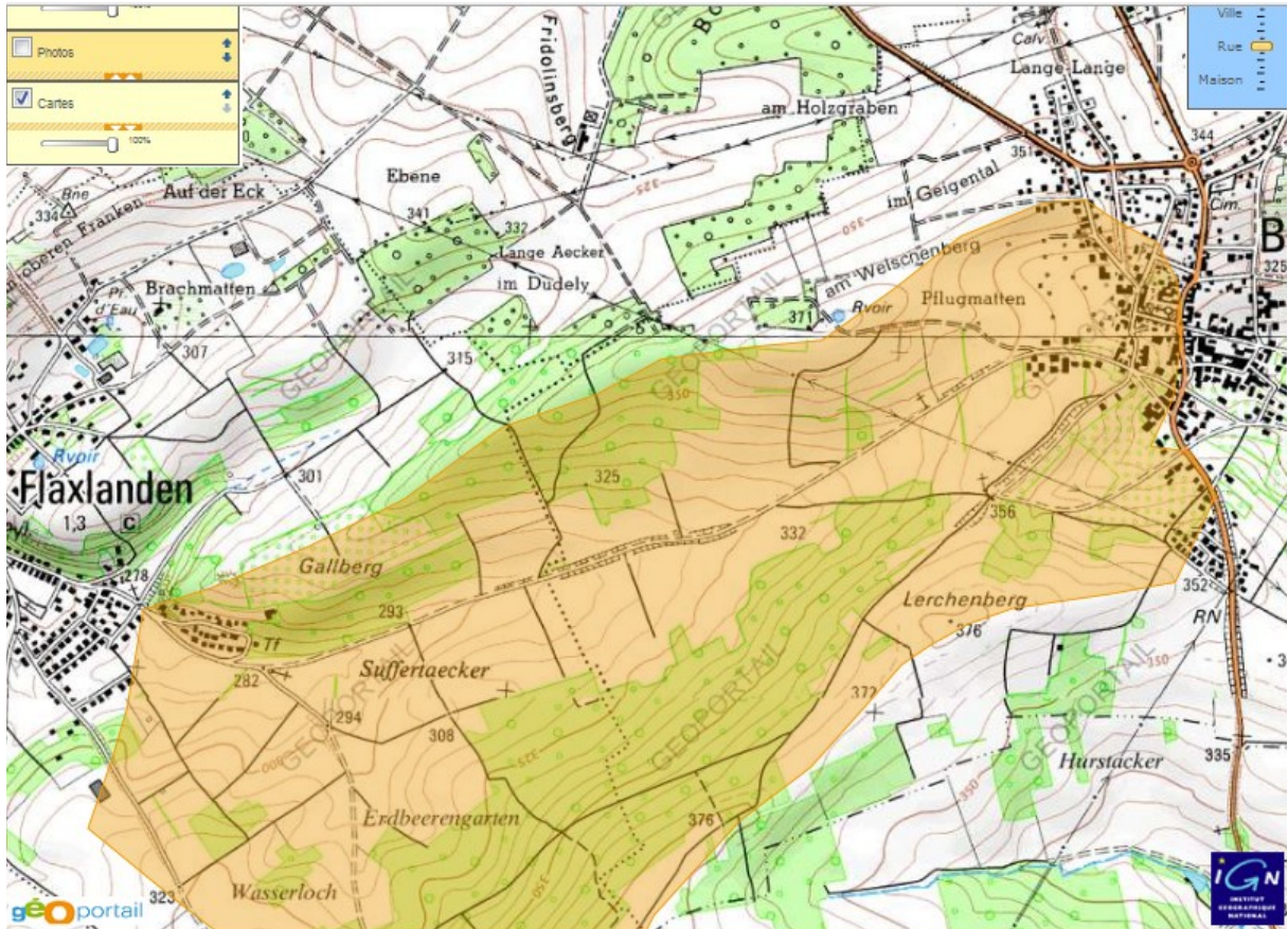
Délimitation du bassin versant : surface = 3.9 km 2
